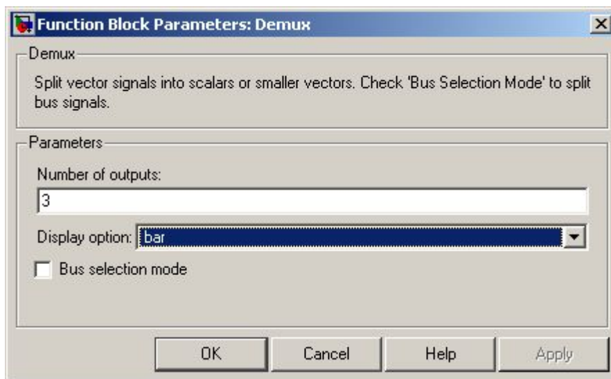
Рис.19.7. Параметры компонента Demux
